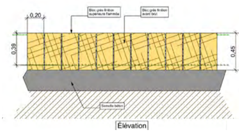
Détail sur escalier Nord
